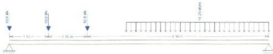
Figura 35 - Posicionamento do trem tipo para cálculo dos esforços cortantes Fonte: Os Autores.
