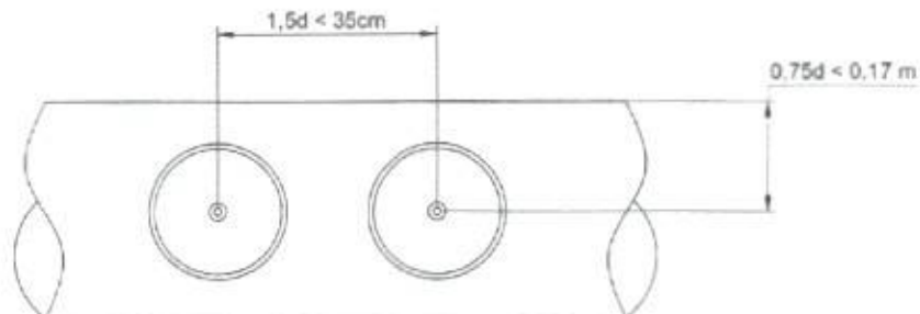
Figura 39 - Verificação dos critérios de distanciamento dos anéis metálicos Fonte: Os Autores.
