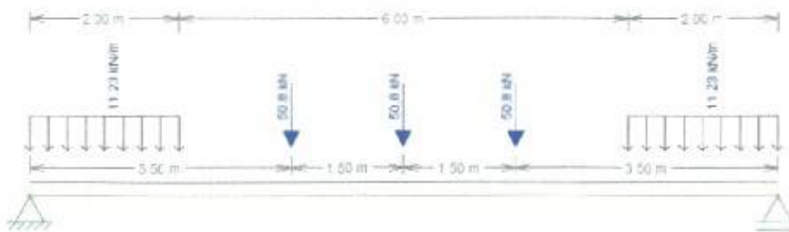
Figura 32 - Posicionamento do trem tipo para cálculo do momento fletor máximo Fonte: Os Autores.
