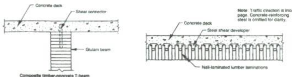
Figura 15 - Tabuleiros compostos de madeira e concreto. Fonte: Calil Junior (2006 p. 45).
