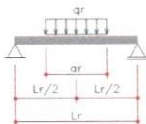
Figura 13 - Posicionamento crítico de uma roda sobre o tabuleiro Fonte: Calli Junior (2006 p. 86).
