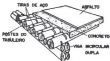
Figura 17 - Tabuleiros compostos de peças roliças de madeira e concreto Fonte: Calil Junior (2006 p. 46).
