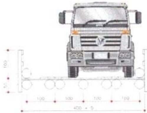
Figura 9 - Posicionamento transversal do veículo-tipo fora do rodeiroFonte: Calli Junior (2006 p. 82).
